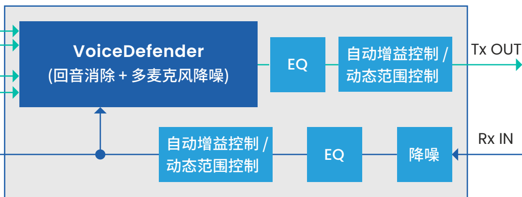
VoiceDefender框图
